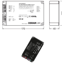
Technische Daten Osramtronic LED Treiber OT 165/170-240/!A0 4DIMLT2 G2 CE
